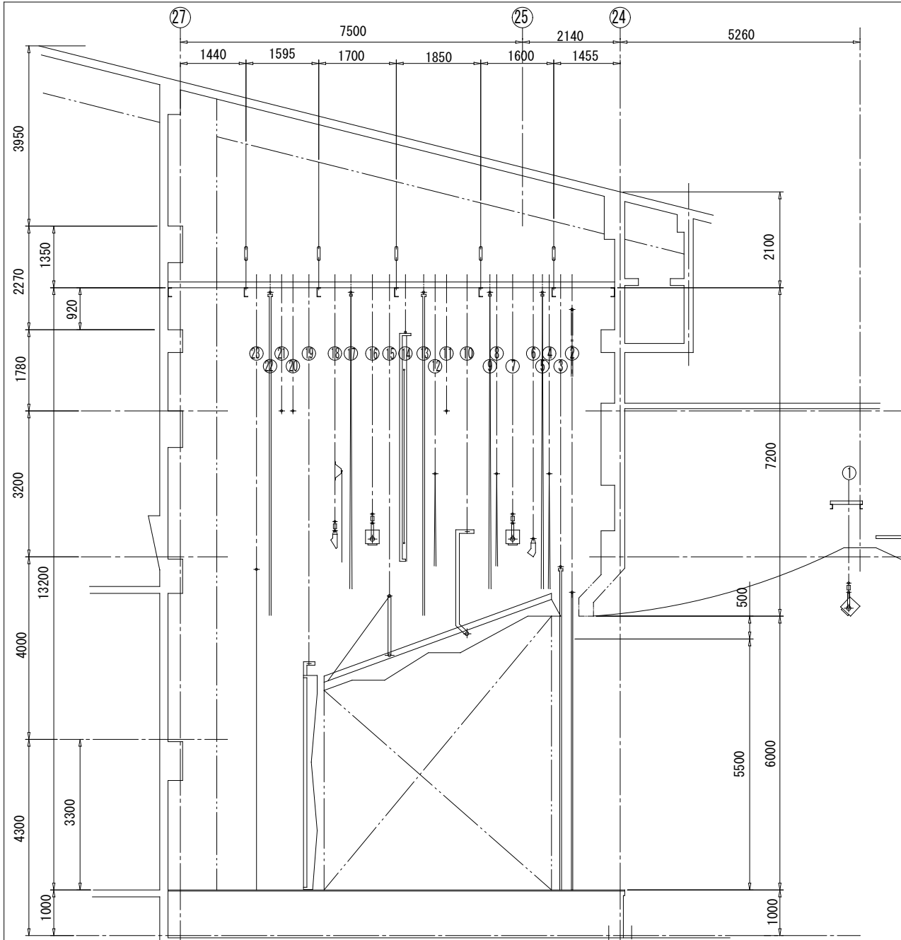
文化ホール舞台吊物装置仕様
